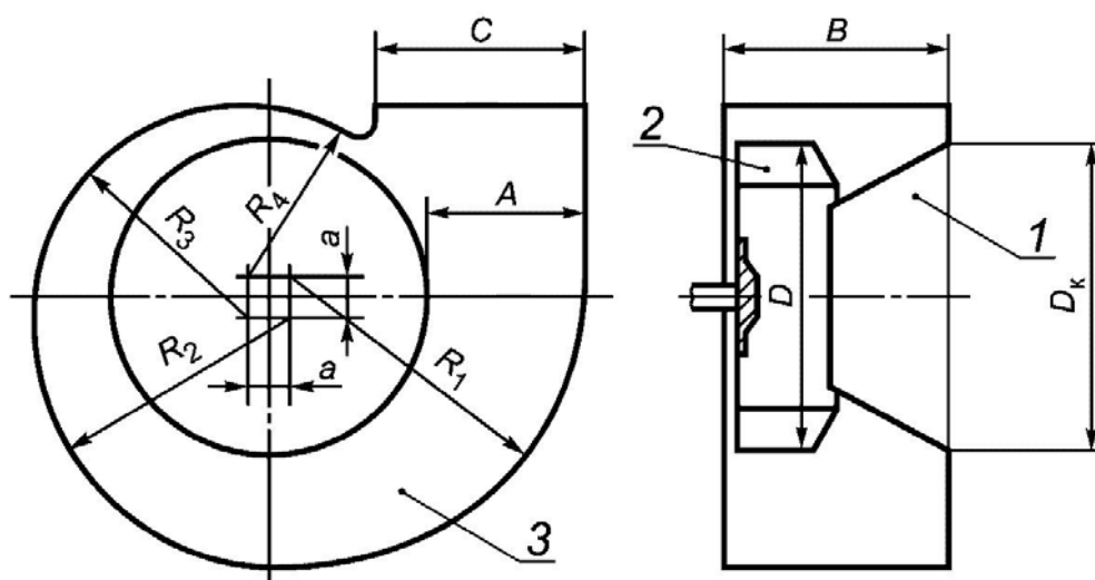
1 - входной коллектор; 2 - рабочее колесо; 3 - спиральный корпус
