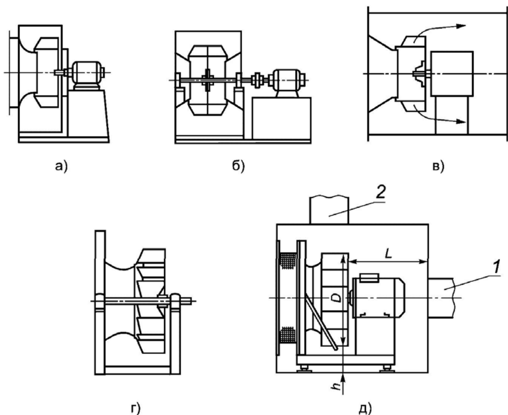
а) односторонний радиальный; б) двусторонний вентилятор; в) прямоточный вентилятор; г) вентилятор - свободное колесо; д) вентилятор в вентиляторном блоке
